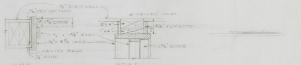
INSIDE DOOR DETAIL
