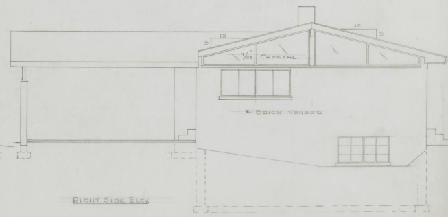
RIGHT SIDE ELEV
